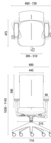
45.101 Giratoria Operativa Brazos 4D-CA Base Up (Nylon)
