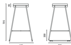
36.814 Spin Stool 705mm
