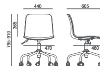
43.003 Giratória
