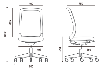
42.101 SR Giratoria Reunión
