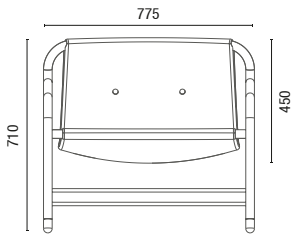
36.906 Sillón Base Fija
