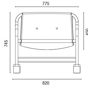
36.906 Sillón Base Esquí
