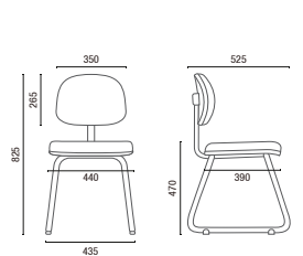
4008 A Secretaria Aproximación
