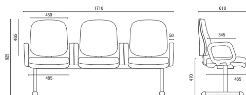
4005 Director Tandem Ancho con Brazo Doble: 2 Puestos - 1140mm 3 Puestos - 1710mm 4 Puestos - 2280mm 5 Puestos - 2850mm
