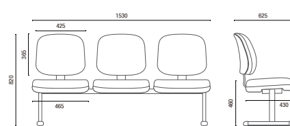
4110 Ejecutiva Tandem Ancho sin Brazo: 2 Puestos - 995mm 3 Puestos - 1530mm 4 Puestos - 2065mm 5 Puestos - 2595mm
