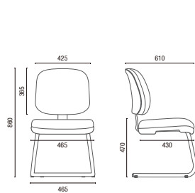
4107 S Ejecutiva Aproximación
