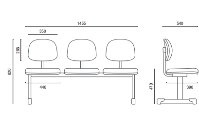
4009 Secretaria Tandem Ancho sin Brazo: 2 Puestos - 950mm 3 Puestos - 1455mm 4 Puestos - 1965mm 5 Puestos - 2470mm
