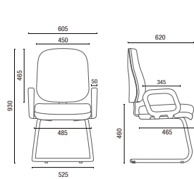
4006 S Director Aproximación
