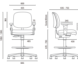
4123 SRE Ejecutiva Stool
