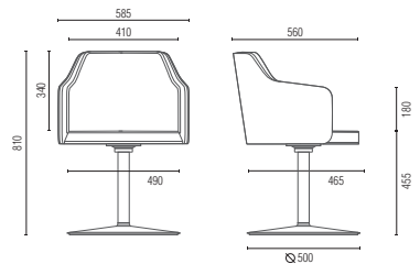
36.272 Poltrona Interlocutor Giratória Base Disco
