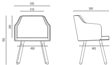
36.174 Poltrona Interlocutor Base Pé Palito
