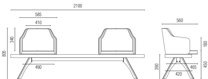
36.075 2L Longarina 2 Lugares
