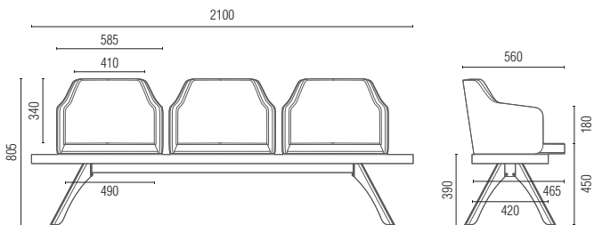
36.075 3L Longarina 3 Lugares
