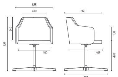
36.172 Poltrona Interlocutor Giratória Base 4 hastes
