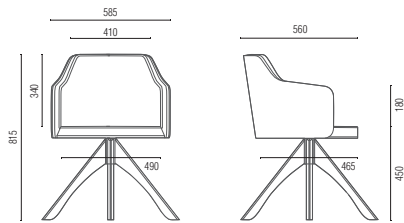
36.074 Poltrona Interlocutor Giratória Base Piramidal
