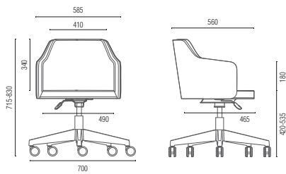
36.071 Poltrona Reunião Giratória Base Twin com Rodízios Opção de Relax
