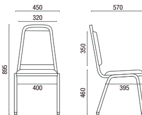
1.001 Empilhável
