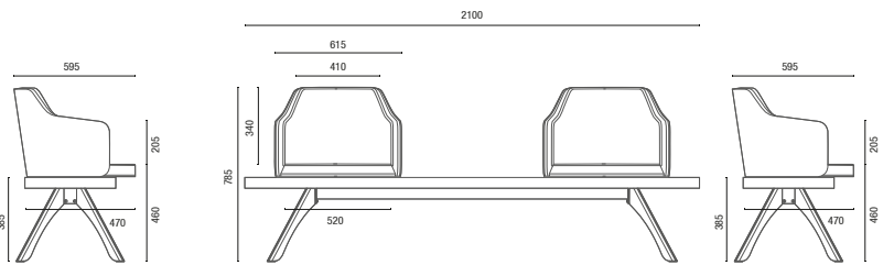
36.075 2L Longarina 2 Lugares
