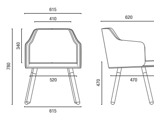
36.174 Poltrona Interlocutor Base Pé Palito
