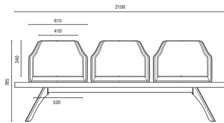
36.075 3L Longarina 3 Lugares
