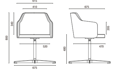
36.172 Poltrona Interlocutor Giratória Base 4 hastes
