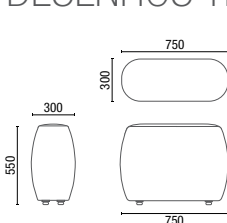
26.201 Braço 300mm
